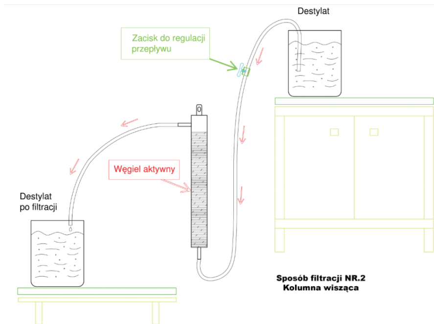
Przykładowy schemat procesu filtracji rys.2
